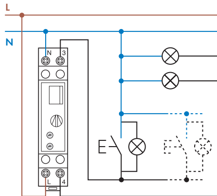
3-проводное соединение
