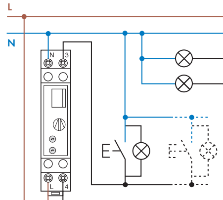
4-проводное соединение
